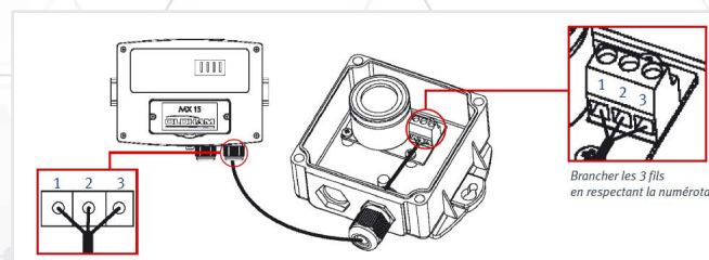
Raccordement d'un détecteur OLC10
