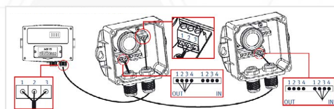
Raccordement de détecteur OLC10TWIN
