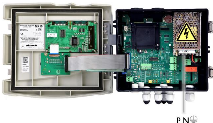
Figure 10 : connexion de l'alimentation secteur
