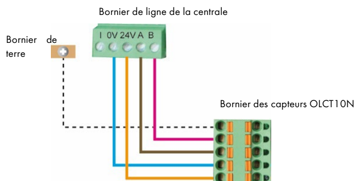
Figure 12: principe de connexion du détecteur numérique sur la ligne de la MX16
