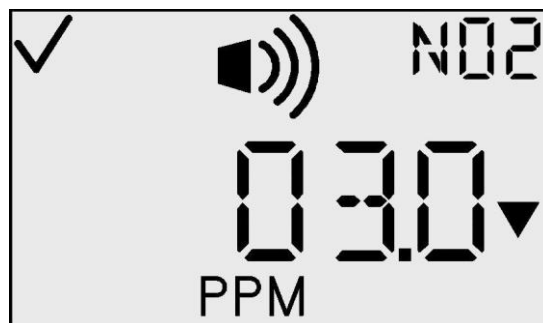
Écran de point de consigne de l'alarme basse
