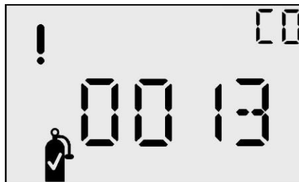
Écran d'échec de l'étalonnage (!)
