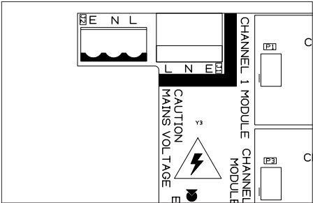
Figure 2.4 Bornes de connexion secteur de la carte PCB du terminal
