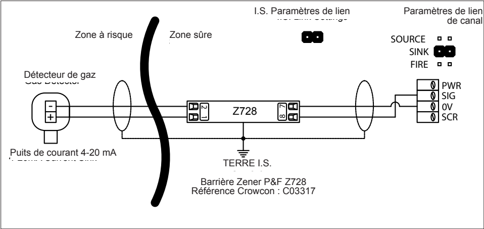
Figure 2.7 Connexions typiques pour un détecteur I.S. 2 fils avec barrière Zener, module d'entrée 4-20 mA/incendie. Réglez le lien du canal sur SINK (voir la Figure 2.5) et la configuration sur DET4-20 SINK (voir la section Présentation du système de menus, pages 25 et 33). Voir les exigences de mise à la terre de la Figure 2.5, page 7.
