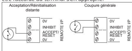
Figure 2.15 Connexions des entrées distantes de coupure/acceptation/réinitialisation
