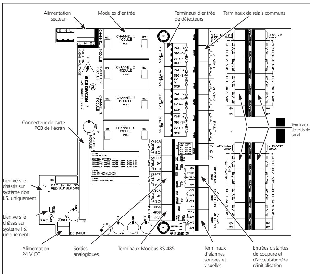
Figure 2.5 Schéma de montage de la carte PCB du terminal
