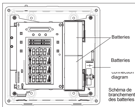
Figure 4.1 Remplacement des batteries
