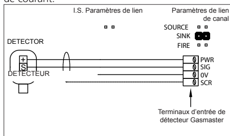
Figure 2.9 Connexions de détecteur à 3 fils, module d'entrée 4-20 mA/incendie
