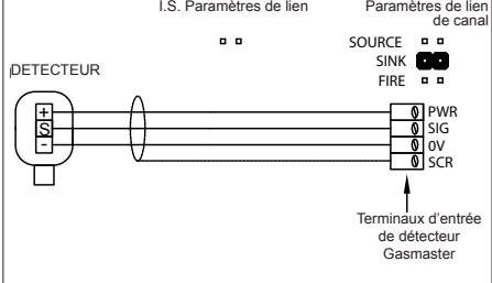
Figure 2.14 Connexions de détecteur de flamme de 4-20 mA à 3 fils, module d'entrée 4-20 mA/incendie
