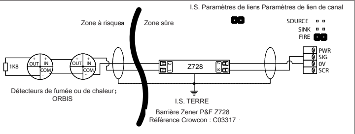
Figure 2.12 Connexions pour les détecteurs d'incendie traditionnels pour zones à risque, module d'entrée 4-20 mA/incendie. Voir les exigences de mise à la terre de la Figure 2.5, page 7.
