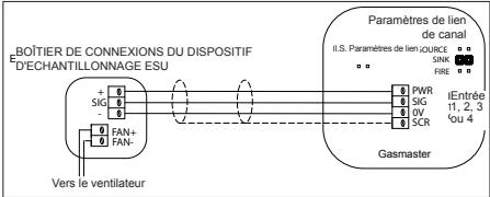
Figure 2.13 Connexions du dispositif d'échantillonnage ESU, module d'entrée 4-20 mA/incendie
