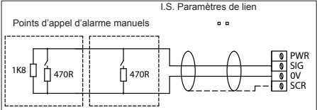
Figure 2.11 Connexions de points d'appel d'alarme manuels, module d'entrée 4-20 mA/incendie
