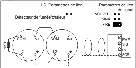
Figure 2.10 Connexions de détecteur de fumée/chaueur, module d'entrée 4-20 mA/incendie
