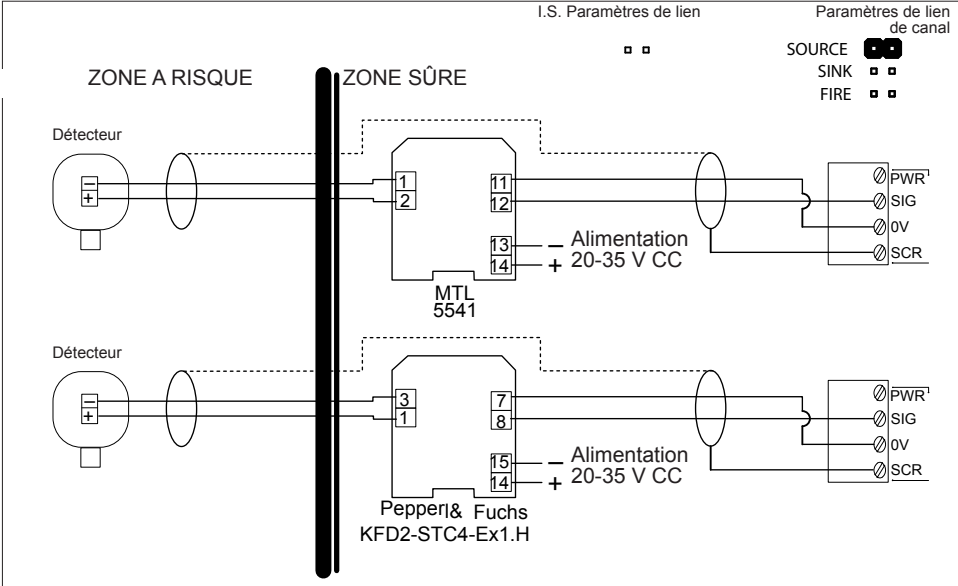
Figure 2.8 Connexions typiques pour un détecteur I.S. 2 fils avec séparateur galvanique, module d'entrée 4-20 mA/incendie. Réglez le lien du canal sur SRCE (voir la Figure 2.5) et la configuration sur DET4-20 SRCE (voir la section Présentation du système de menus, pages 25 et 33).
