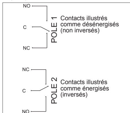
Figure 2.17 Les contacts du Gasmaster pour tous les relais sont identifiés sur la carte PCB du terminal.
