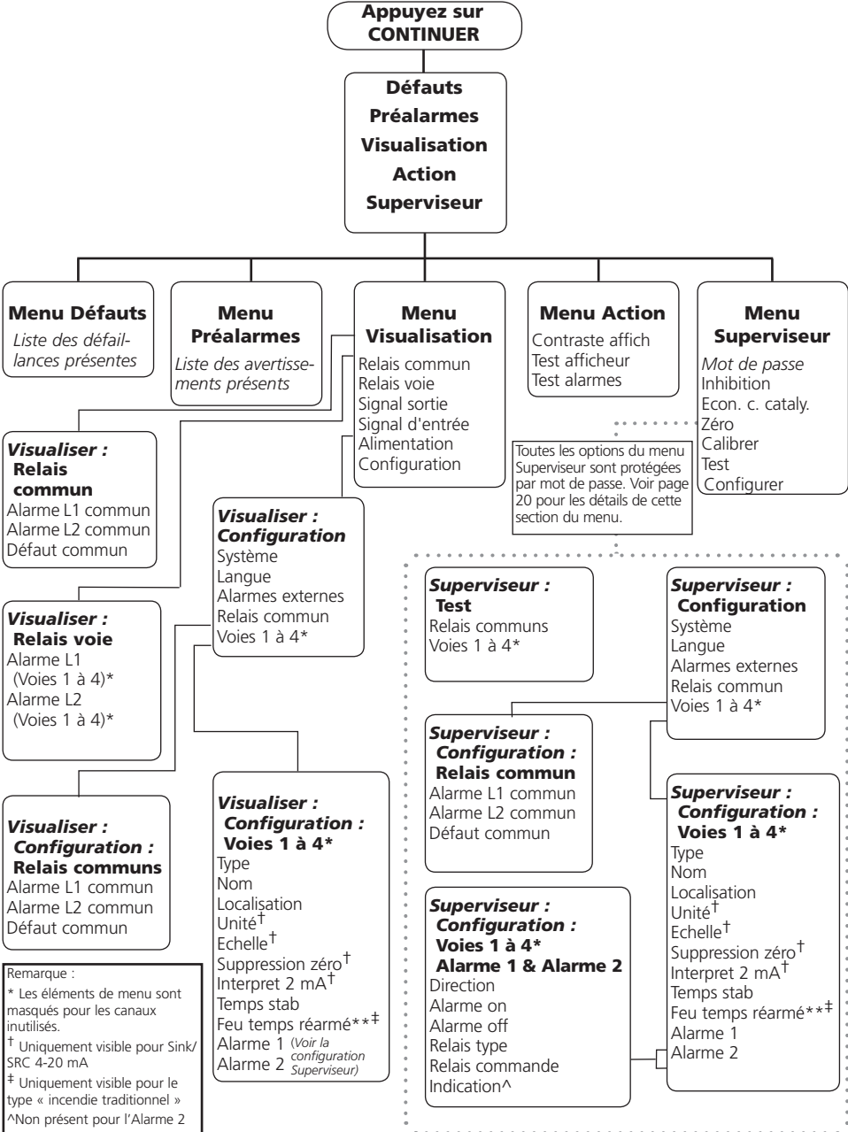
Figure 3.5 Présentation du système de menus du Gasmaster
