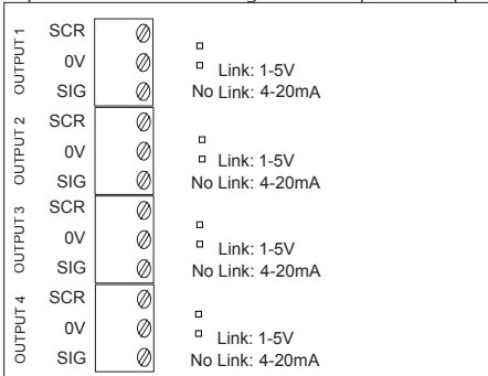
Figure 2.18 Terminaux de connexion des sorties analogiques du Gasmaster
