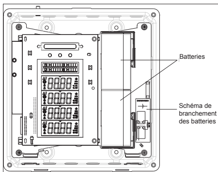
Figure 2.2 Plaque du châssis du Gasmaster avec carte PCB de l'écran et batteries.
