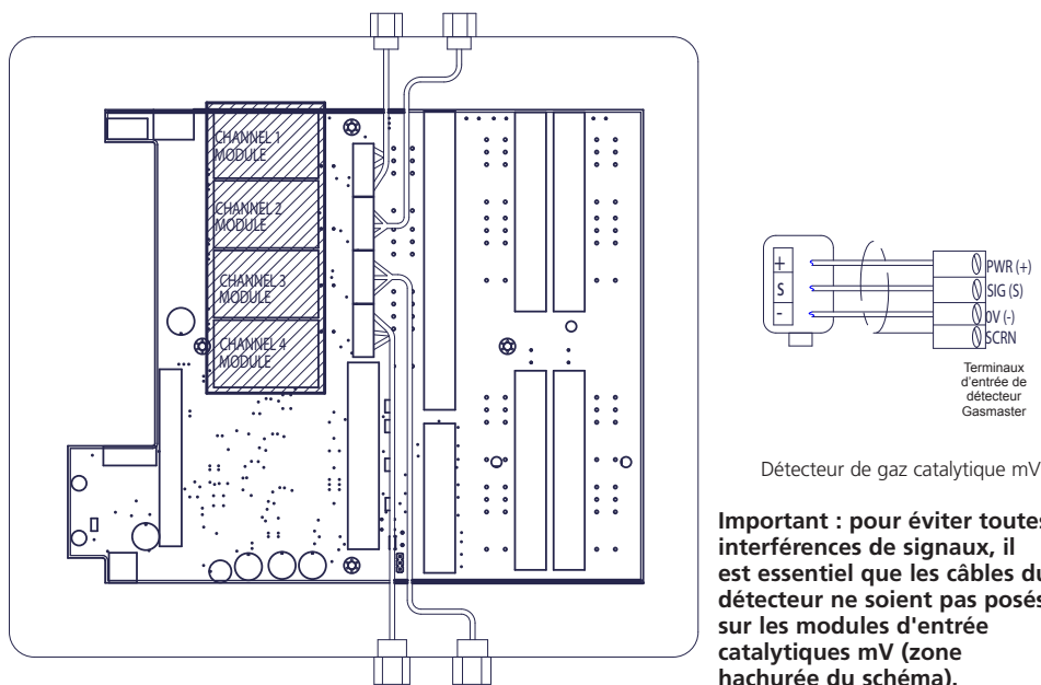
Figure 5.1 Connexions pour détecteurs de type catalytique mV. Module d'entrée catalytique mV.
