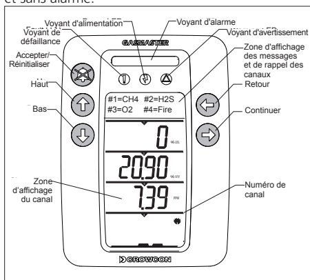
Figure 3.1 Panneau d'affichage et boutons de commande
