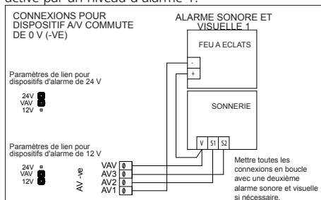
Figure 2.16 Connexions pour l'entraînement AV
