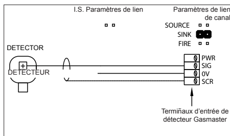
Figure 2.6 Connexions de détecteur à 2 fils, module d'entrée 4-20 mA/incendie
