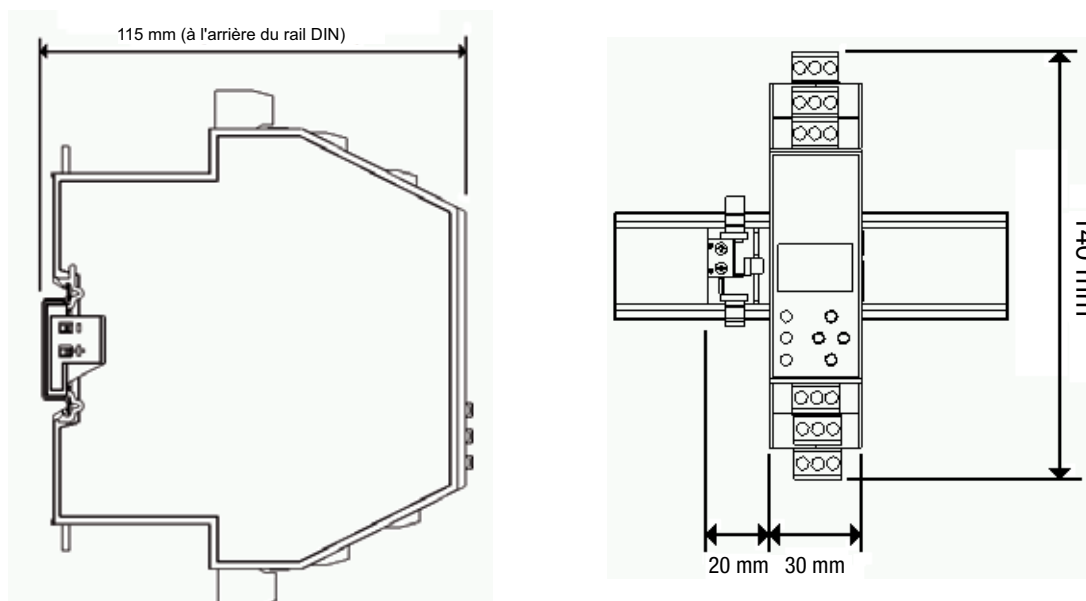
Schéma des cotes générales
